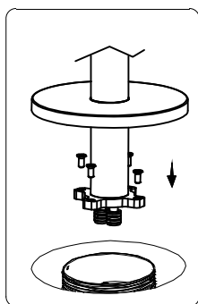
4. Установите трубку смесителя (поз. 1) на монтажный блок, выровняйте направление. При необходимости поверните излив на 360° перед окончательной фиксацией.
