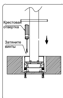
6. Затяните крепежные винты с помощью крестовой отвертки.
