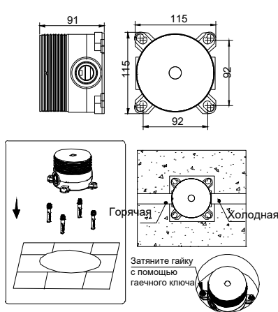
1. Монтаж встраиваемого блока
