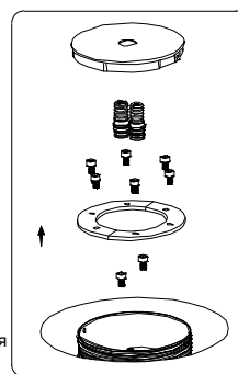
2. Снимите защитный кожух с монтажного блока.
