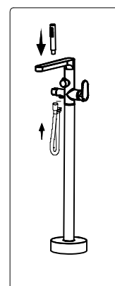
7. Соедините душевой шланг и лейку. Откройте вентили и проверьте систему на герметичность.
