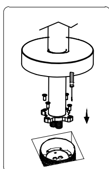
5. Установите все элементы в указанном порядке. Вставьте винты (4), как показано на рисунке.
