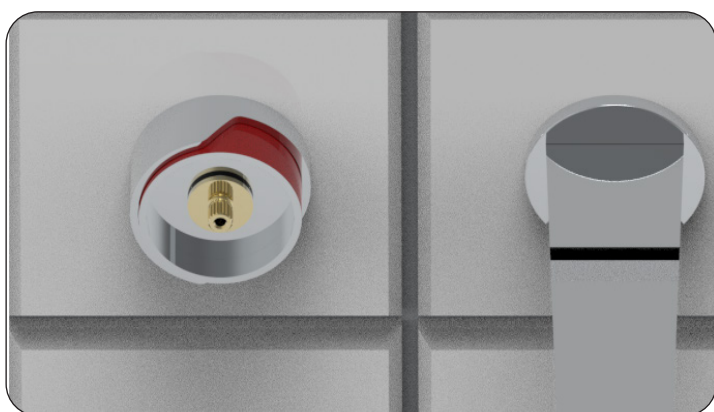
Positionnement de la bague pour les croisillons Zoom / Positioning the ring for the Zoom braces
