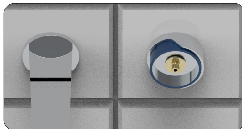
Positionnement de la bague pour les croisillons Zoom / Positioning the ring for the Zoom braces
