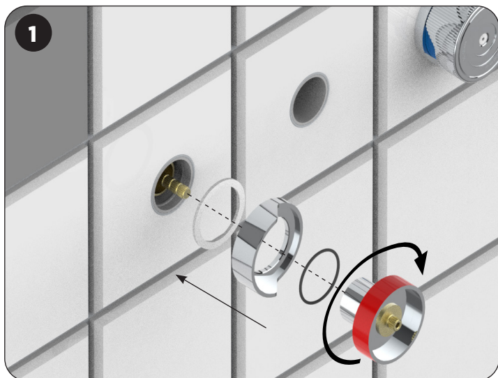
Positionnement de la bague pour les croisillons Zoom / Positioning the ring for the Zoom braces
