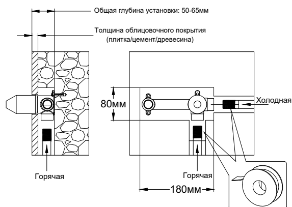
Встраиваемый корпус смесителя без блока
