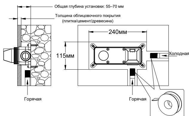
Встраиваемый корпус смесителя с блоком
